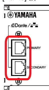
配备 Dante 的 XMV 型号的 [Dante] 接口
