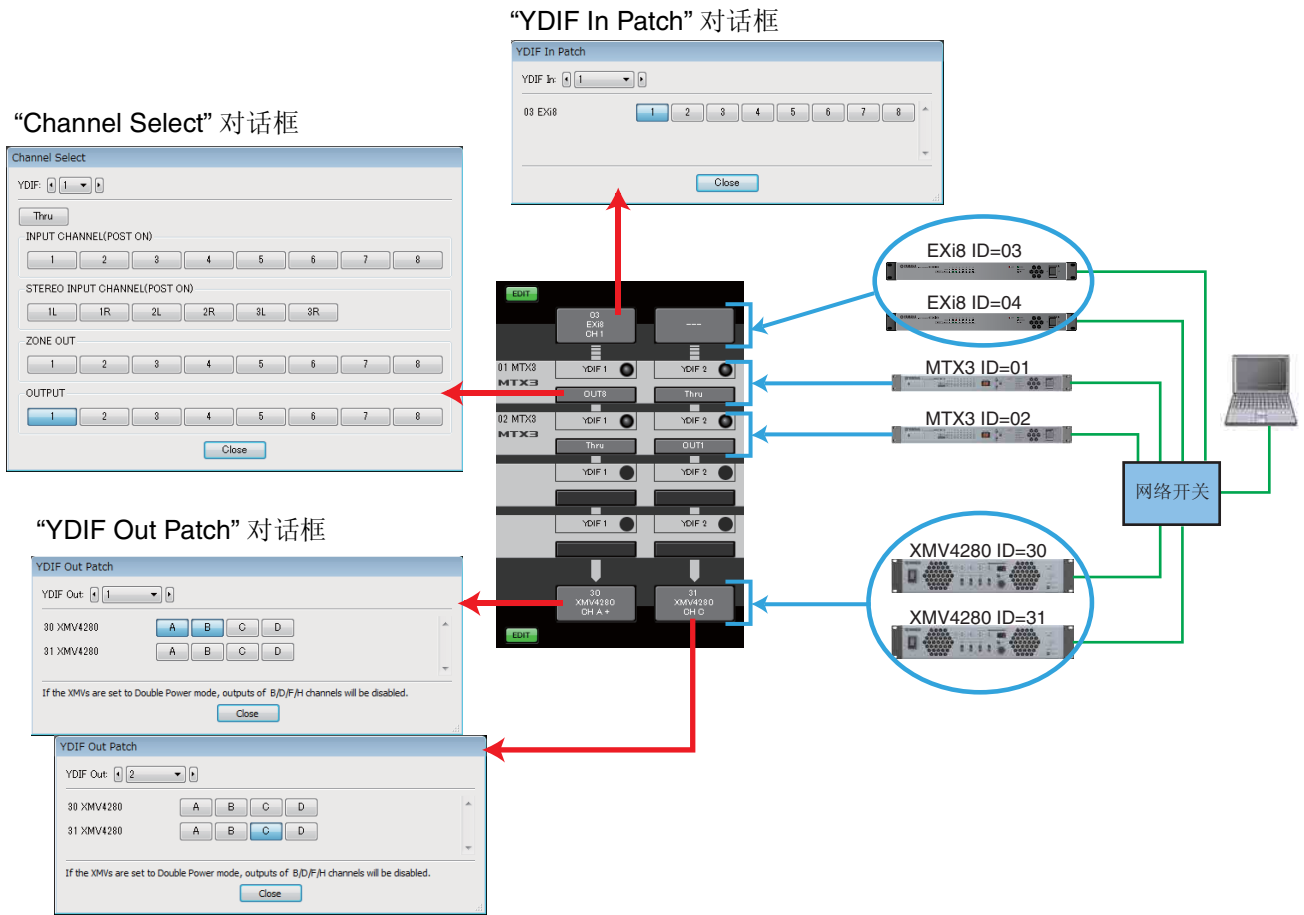
采用上述设定的 YDIF 信号流
