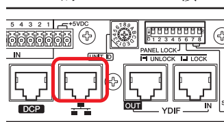
MTX3 的 NETWORK 接口
